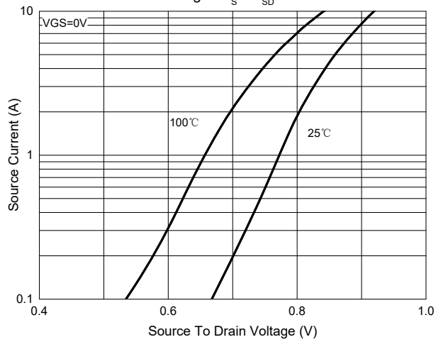
Fig.9 - I_s - V_{SD}
