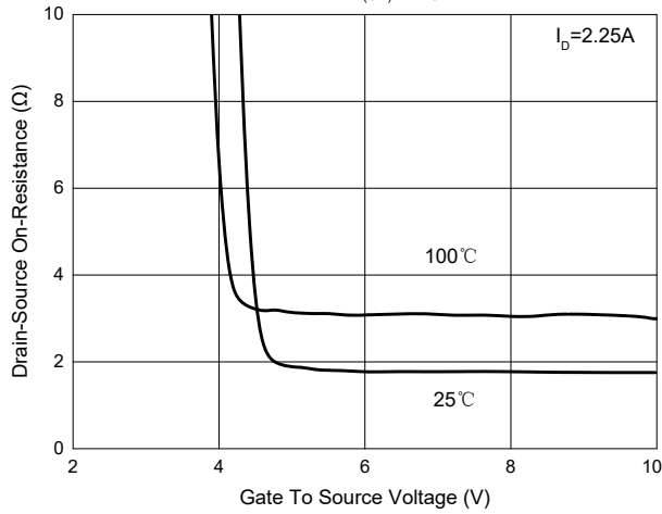
Fig. 3 - R_{DS(ON)} - V_{GS}
