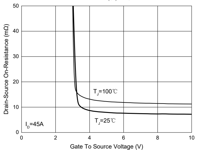
Fig. 6 - R_{DS(ON)} - V_{GS}
