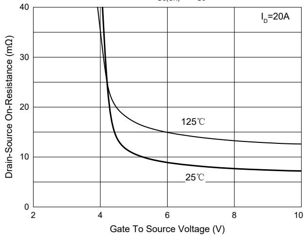
Fig. 3 - R_{DS(ON)} - V_{GS}
