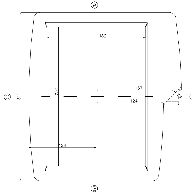
Oberschale (Außenansicht)
