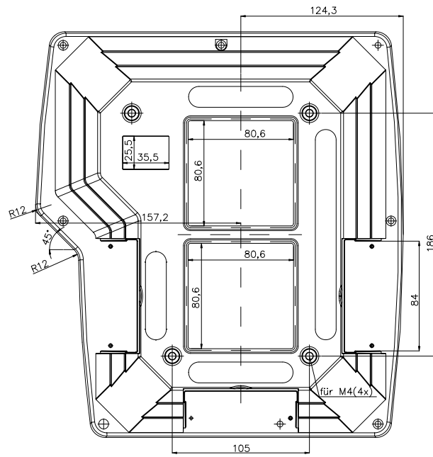
Unterschale (Außenansicht)
