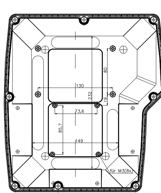
Unterschale (Innenansicht)
