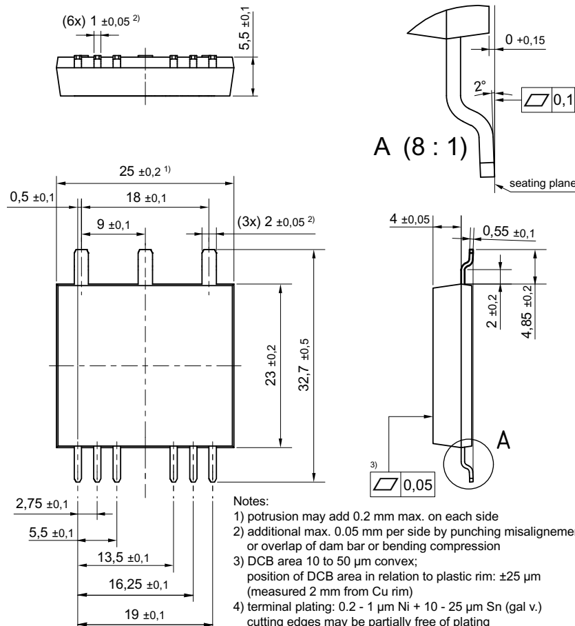
X030a SMPD-B
