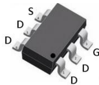
SOT-23-6
