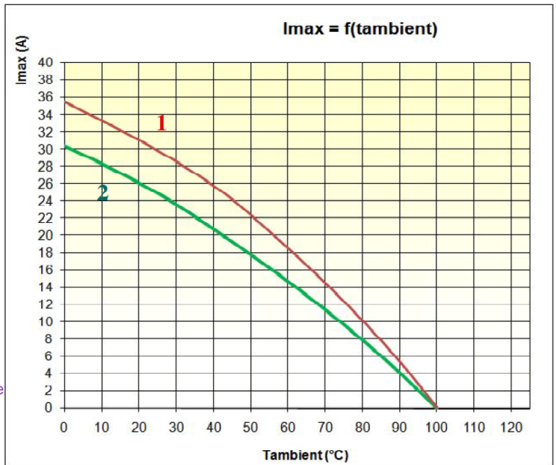
Fig. 2 Courbes thermiques & Choix dissipateur thermique / Thermal curves and heatsink choice
