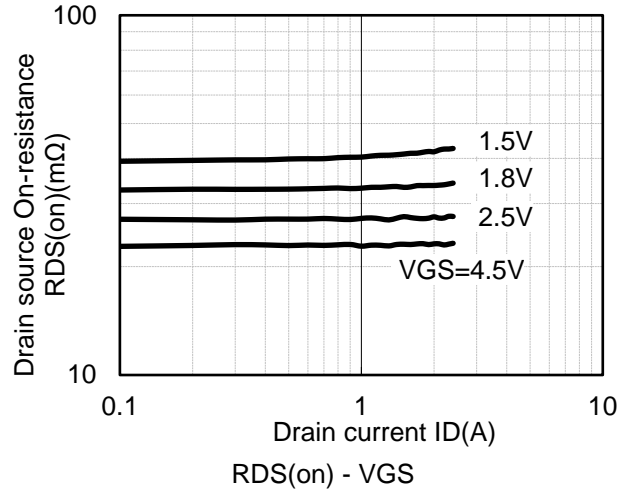
RDS(on) - ID
