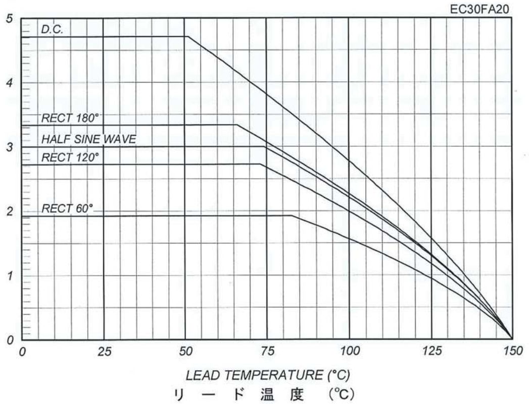
平均順電流 - リード温度定格 AVERAGE FORWARD CURRENT VS. LEAD TEMPERATURE
