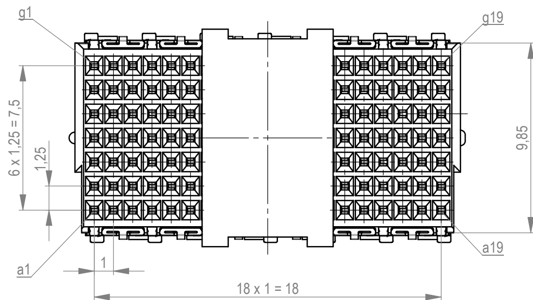
Leiterplatten-Layout Vorschlag PCB-layout proposal
