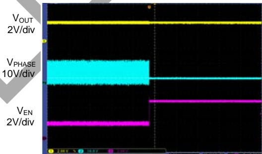
MODE Transition CCM to DEM
