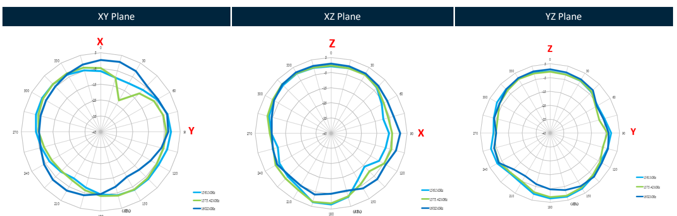
1602MHz
