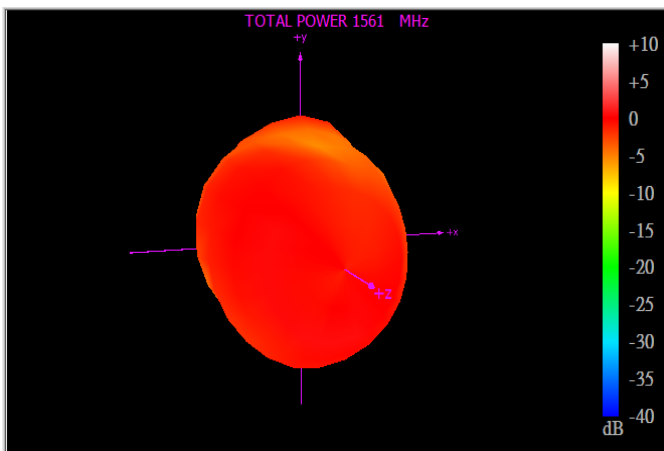
1561MHz
