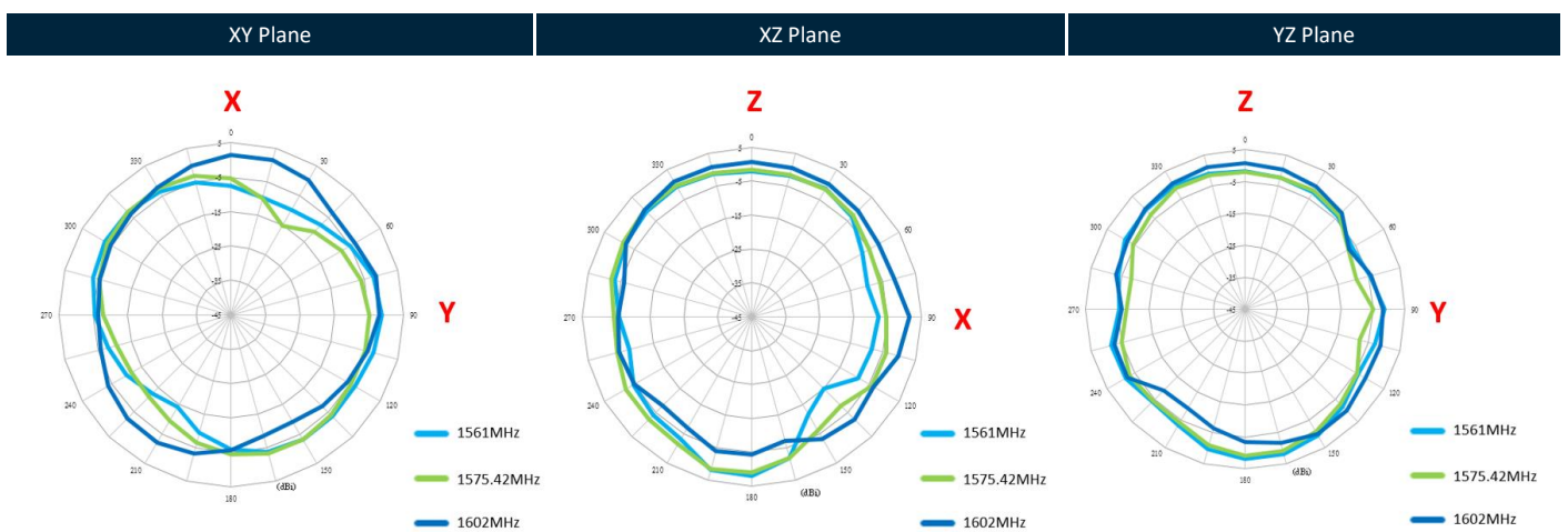
1602MHz
