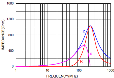
AFBC-Q0805G-471
