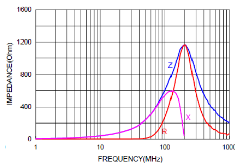
AFBC-Q0805G-601
