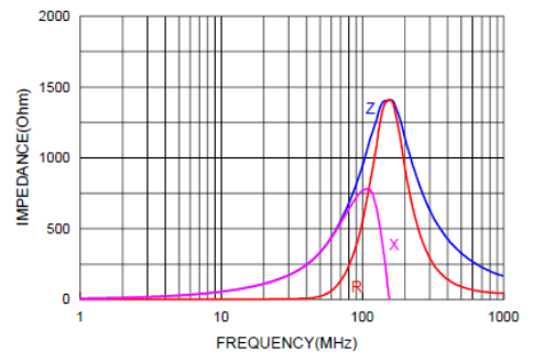
AFBC-Q0805G-102
