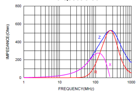
AFBC-Q0805G-301
