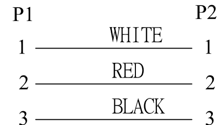
接线示意图
