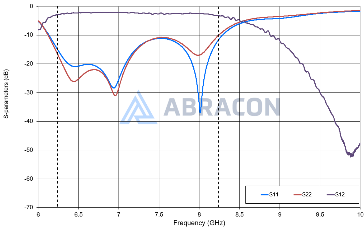
S-parameters
