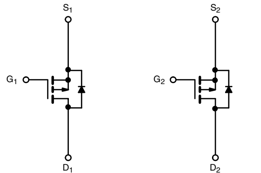
P-Channel MOSFET
