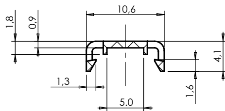
SEZIONE A-A
