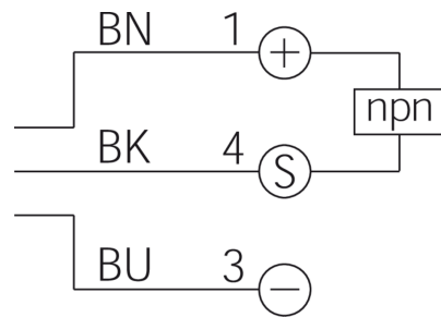
1) LED 2) Schlüsselweite 17 mm BK: schwarz BN: braun BU: blau
