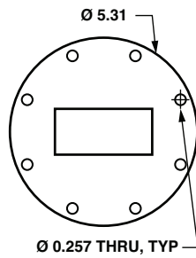
WR284 (UG-584/U)
